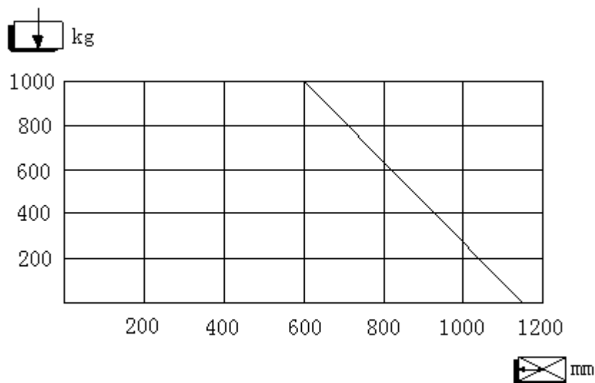
Lastdiagramm
